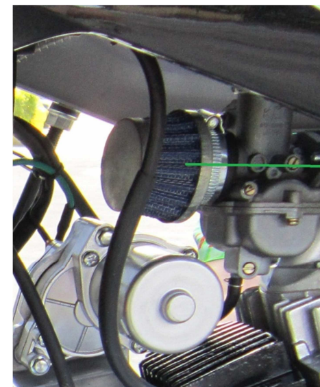
регулирующая гайка
