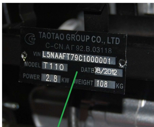
Номерная табличка
