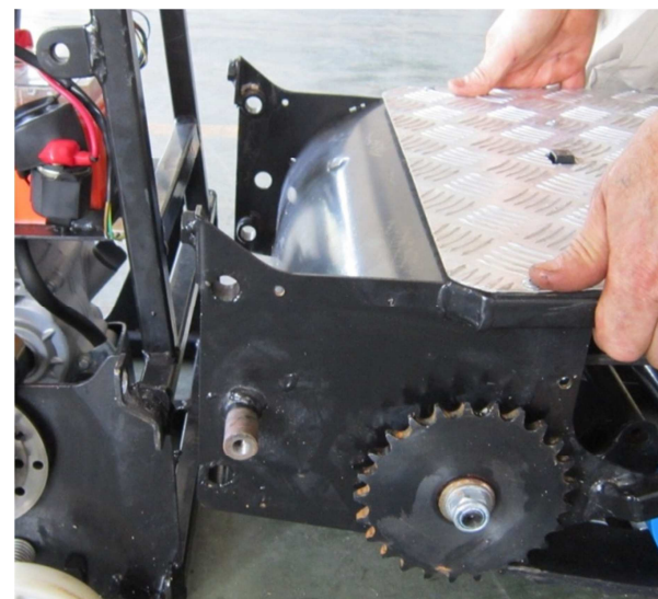
14. Вытаскиваем гусеничный блок из направляющих.
